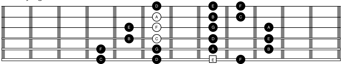
FM13#11
